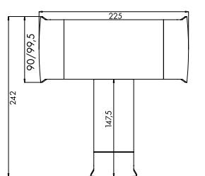
212,5/252,5 ingombro totale con contenitore di servizio total dimension with service unit 90/99,5 176/214
